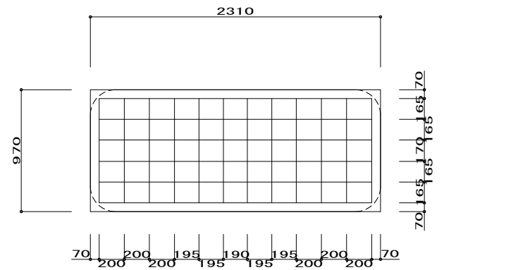
ベース配筋図 1/30
