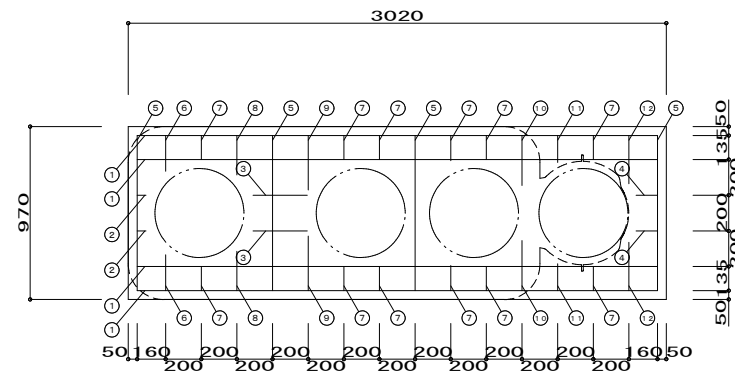
スラブ配筋図 1/30
