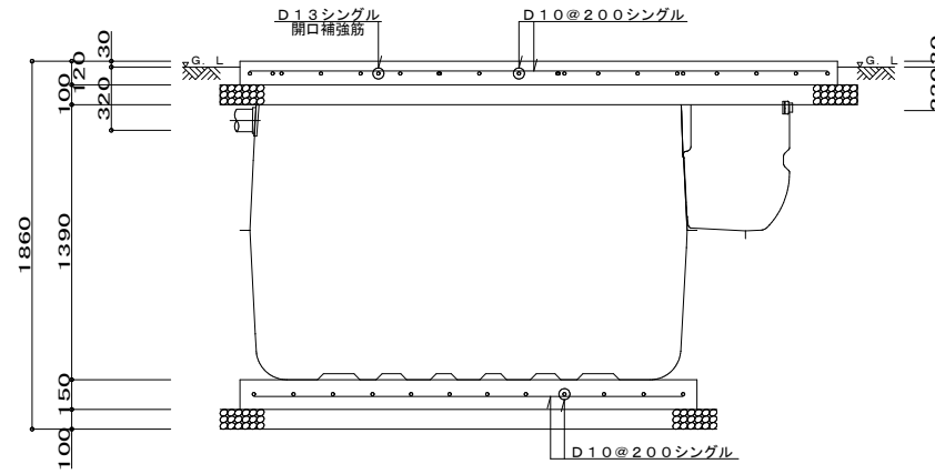
軸方向断面配筋図 1/30
