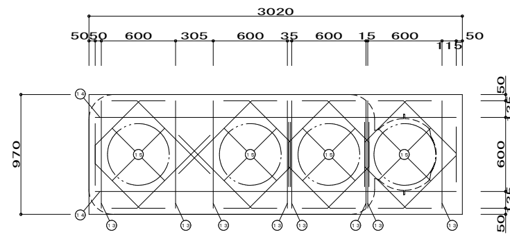
スラブ開口配筋図 1/30
